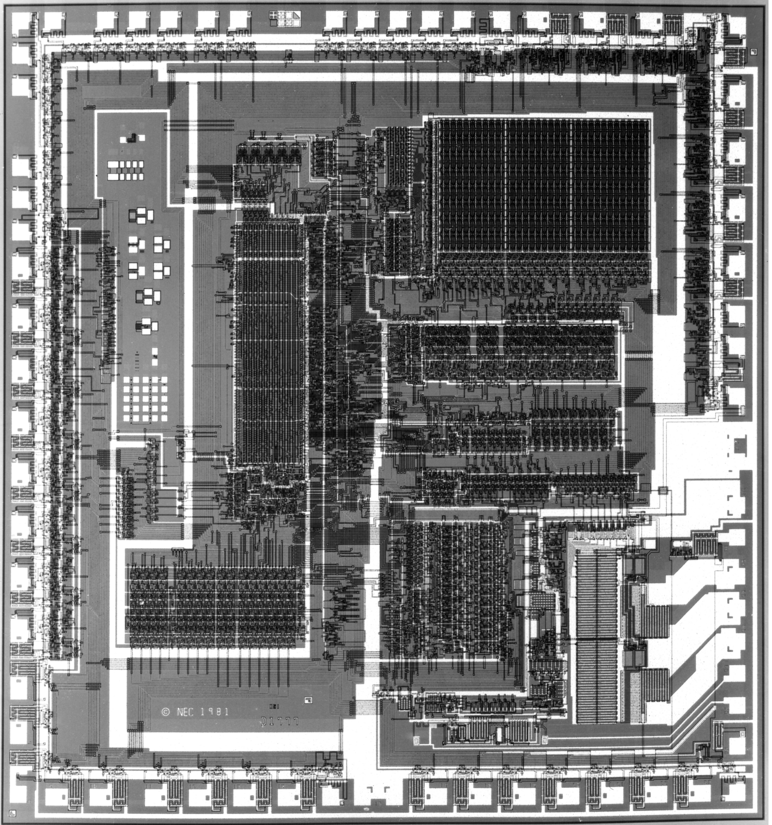
μPD1777/1770 Die
