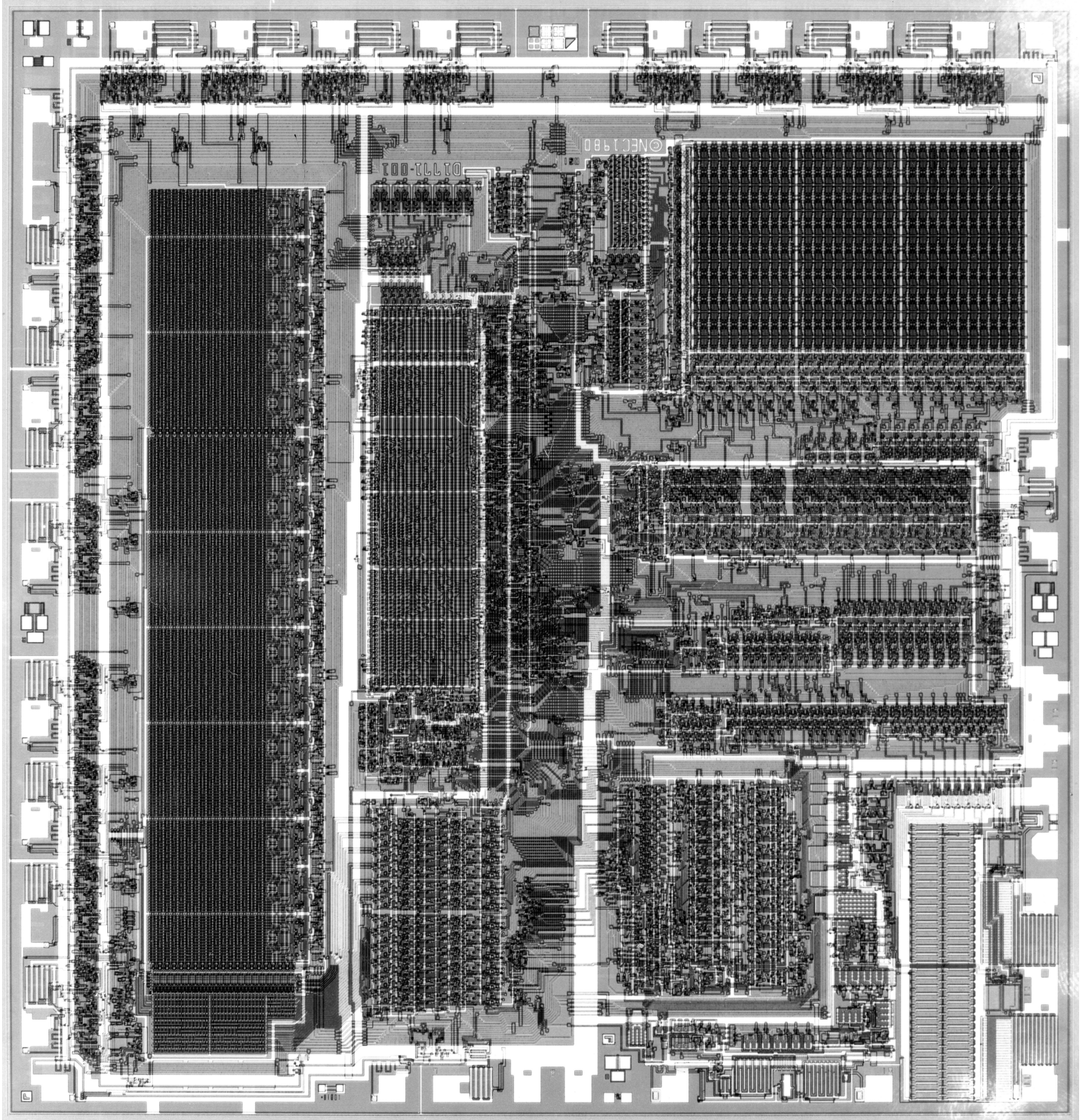
μPD1771 Die
